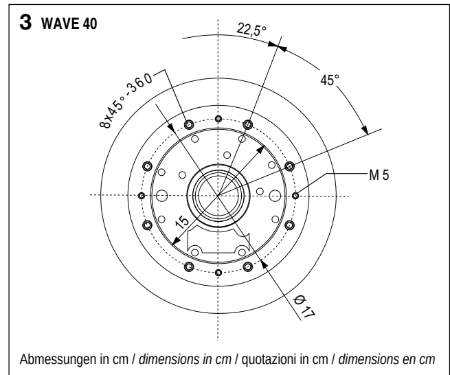
Schema di foratura WAVE 40 Fig. 3.
